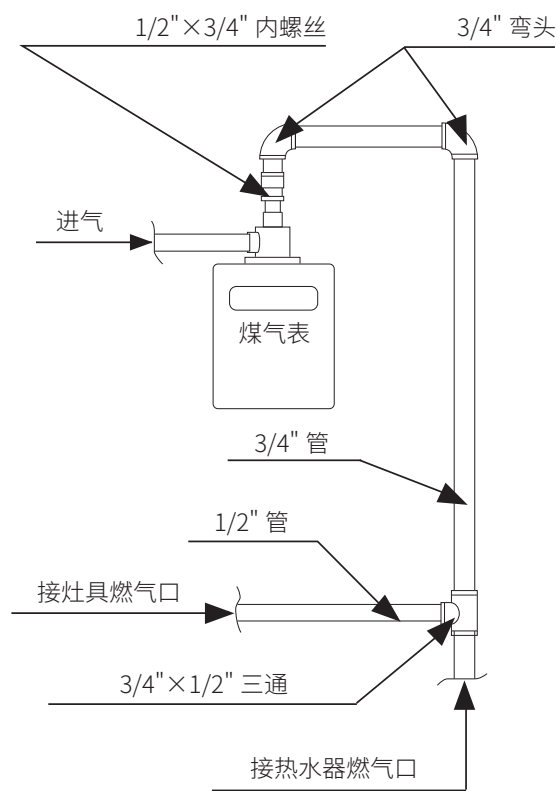
煤气表出口燃气管装接法
