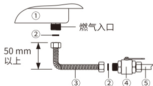
①燃气灶 ②密封圈 ③波纹软管 ④阀门 ⑤燃气管（硬管）
