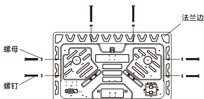
① 将可调螺钉拧入底壳箭头指示位置。
