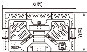
② 螺钉按实际开孔尺寸调节对应的X(宽)和Y(深)的尺寸，用螺母固定。
