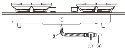
①燃气灶 ②波纹软管 ③阀门 ④燃气配管（硬管）
